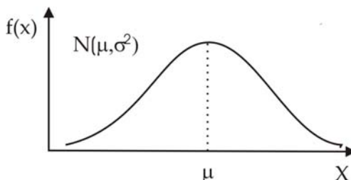
Slika 2. Gausova funkcija
