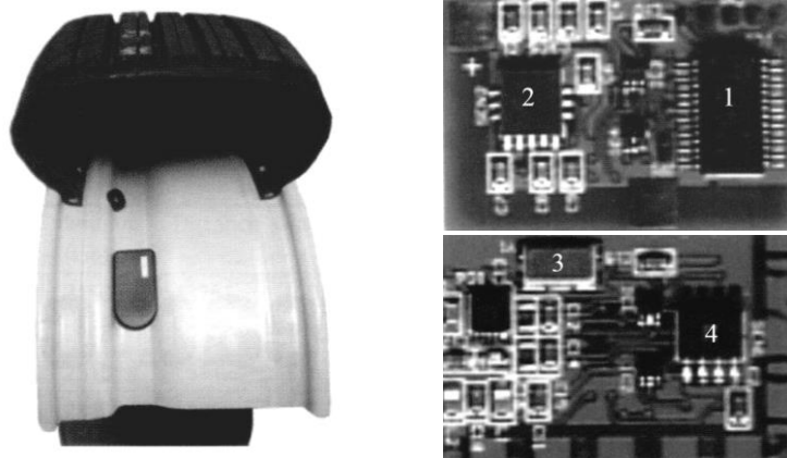
Sl. 5. Položaj davača na naplatku i njegov izgled sa pripadajućim komponentama (1. mikroprocesor, 2. G senzor, 3. transmiter, 4. senzor pritiska)[1], [2]
