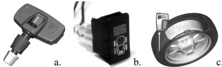
Sl. 6. Varijanta zasebnog sistema za praćenje stanja pritiska u pneumaticima (a. davač na ventilu pneumatika, b. kontrolna jedinica, c. davač na naplatku sa izgledom kontrolne jedinice)[1], [2]
