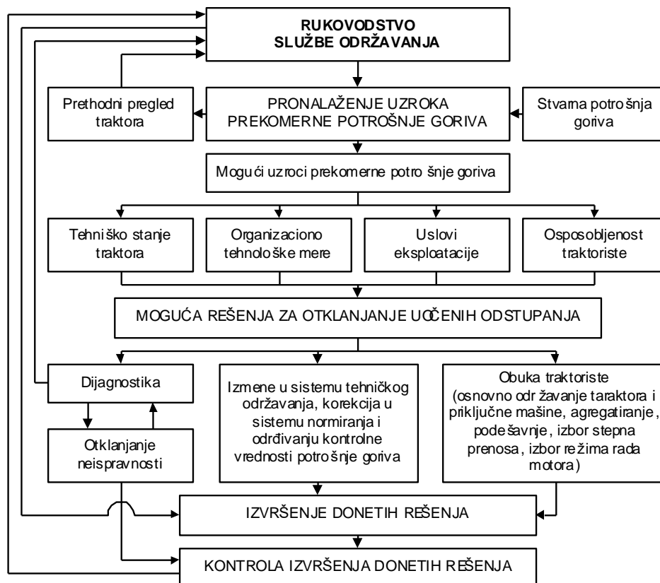
Sl. 5. Šema sistema kontrole uzroka koji dovode do prekomerne potrošnje goriva i mere za njihovo otkrivanje
