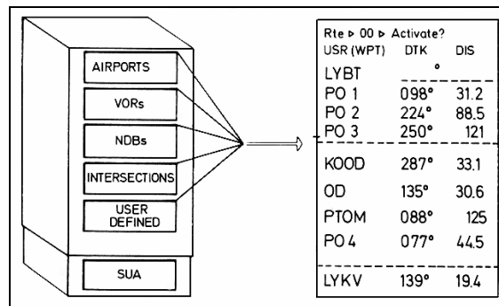
Слика 4. Навигацијска база података и дефинисање корисничке тачке омогућавају брзо креирање маришуте лета
