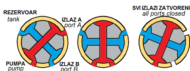
Slika 7. Obrtno klizni razvodnik sa dva izlaza.
