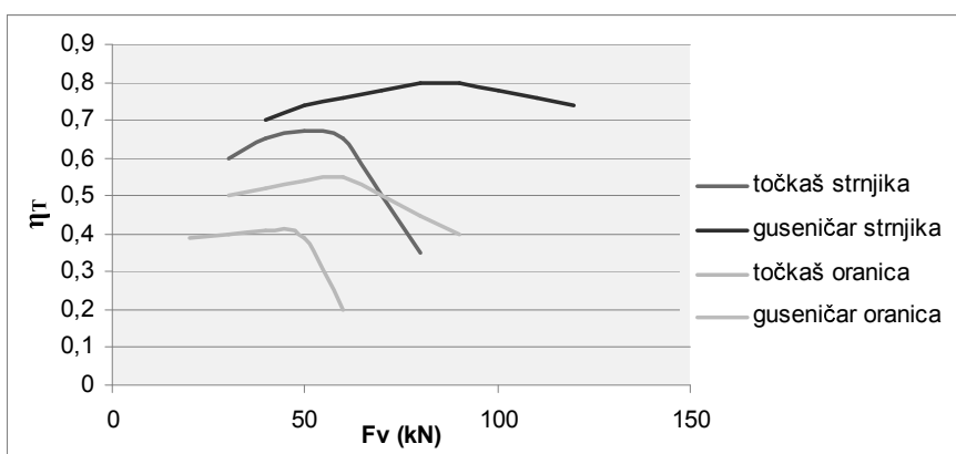
Sl. 7. Vrednosti koeficijenat korisnog dejstva traktora
