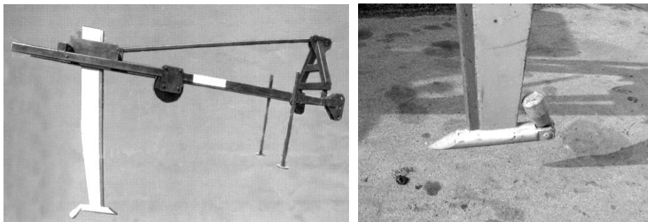
Sl. 2. Drenažni plug DP-4
