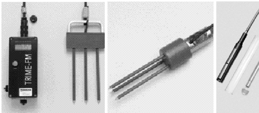
Slika 4. Trime FM-3 tropinska sonda, sonda za bušotine sa tri pina i adapterom i cevna sonda, tankozidna cev i čep
