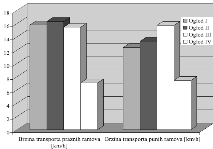
Sl. 14 Transportne brzine praznih u punih ramova
