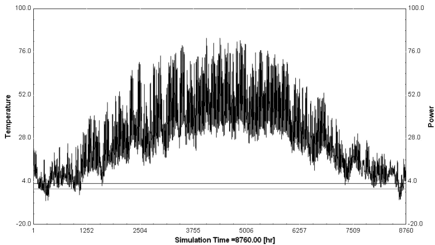
Slika 2. Časovni profili temperature unutar objekta tokom godine bez sistema za grejanje
