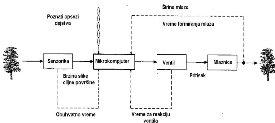
Sl. 1. Princip funkcionisanja senzorski upravljane aplikacije
