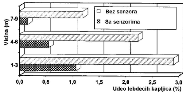
Sl. 2. Smanjenje drifta lebdećih čestica u zavisnosti od visine
